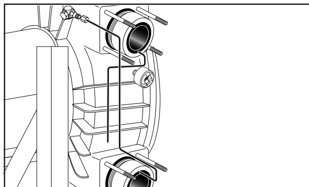
Rys. 25 Rurka odpowietrzająca
