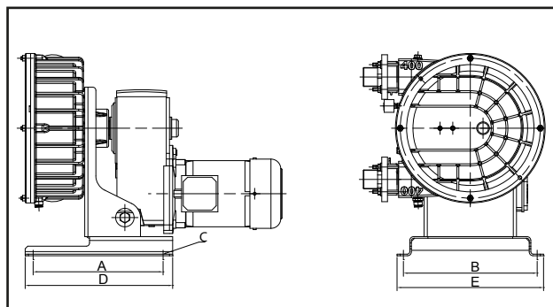
Rys. 10 Wymiary podstawowe
