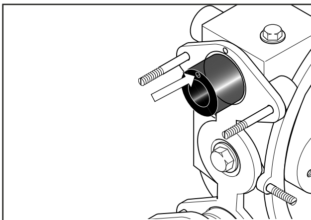
Rys. 20 Położenie otworu próżniowego IP 100/200
