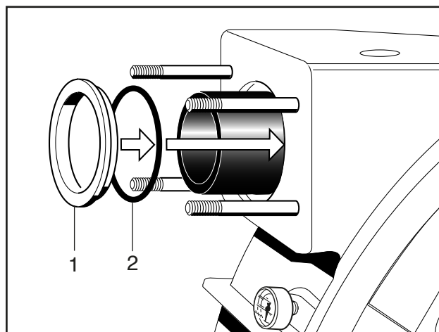
Rys. 34 Montaż pierścienia stopniowanego
