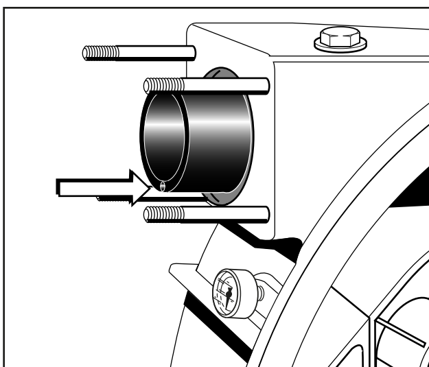
Rys. 21 Położenie otworu próżniowego IP 400-800
