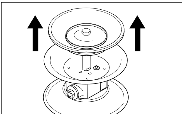
Rys. 12: Wyciągnąć tłoczysko.
